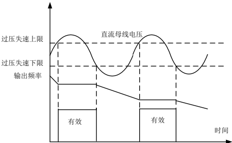
图 7-18 过压失速
