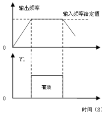
图 7-13 输入输出平衡
