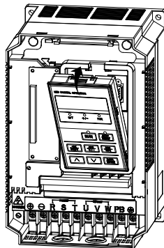
图 2-5 键盘安装图示
