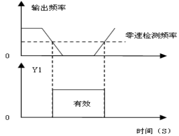
图 7-20 频率零速检测
