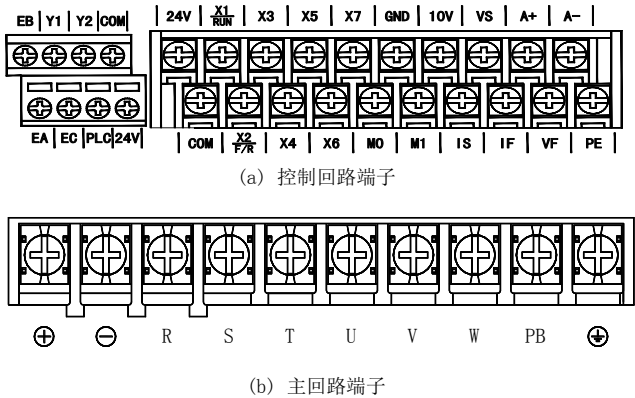
图 1-5 控制回路端子和主回路端子
