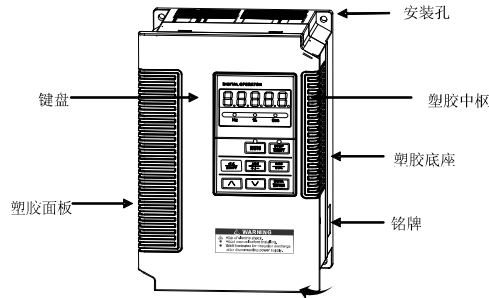
图 1-4 HGD303 系列变频器外形及部件
