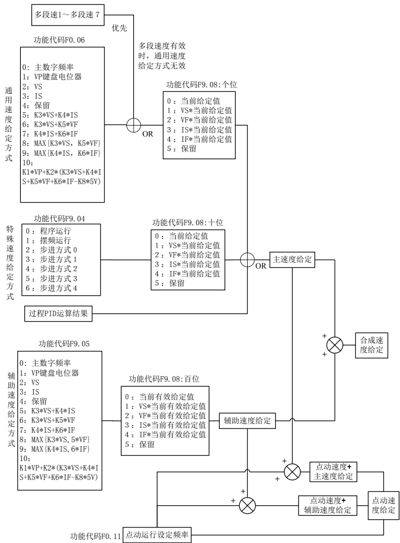
图 1-1 速度输入方式示意图
