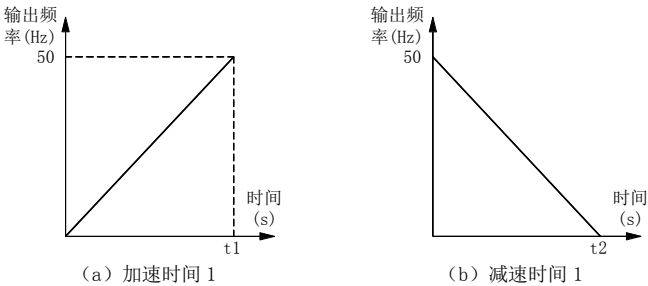
图 7-4 加减速时间
