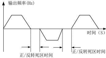
图 7-6 正/反转死区时间示意图
