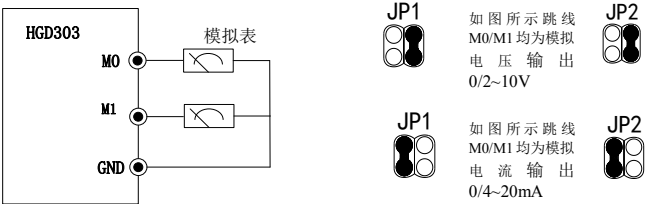
图 3-15 模拟输出端子配线
