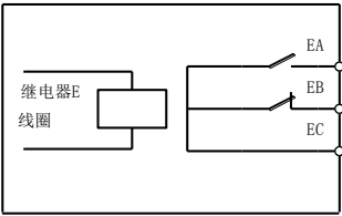
图 7-9 继电器触点
