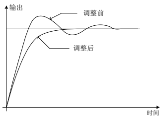
图 7-27 抑制输出超调
