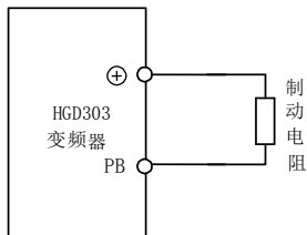
图 11-1 制动电阻的连接
