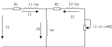
图 8-1 三相异步电动机等效电路
