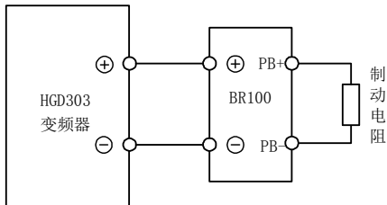
图 11-2 制动单元的连接
