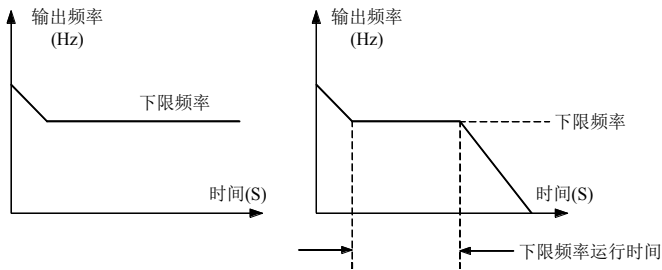
图 7-24 下限频率控制示意图
