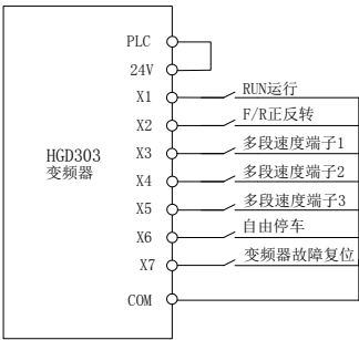
图 7-1 端子控制接线
