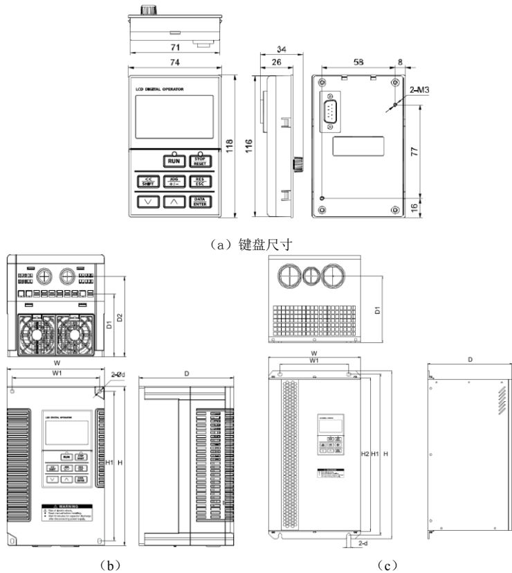
图 2-1 HGD303 系列开环矢量控制变频器和键盘外形尺寸图
