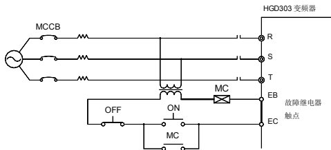
图 3-4 接入输入断路器
