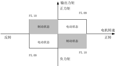
图 7-30 电动/制动力矩电流限定
