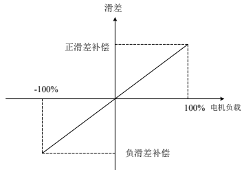
图 8-3 滑差补偿
