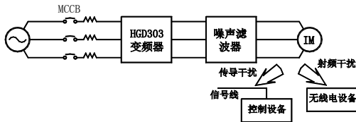
图 3-7 输出侧安装噪声滤波器
