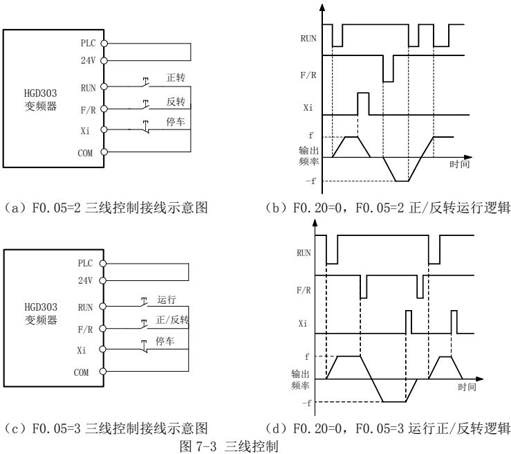
图 7-3 三线控制
