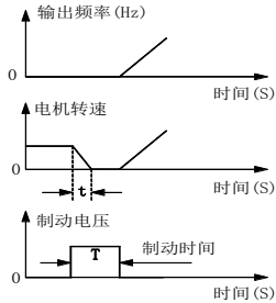
图 7-22 启动直流制动过程
