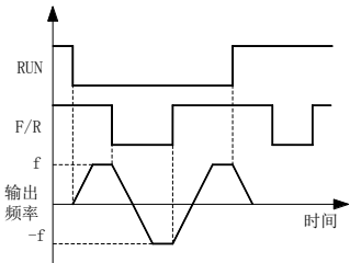
（b）F0.20=0，F0.05=0 运行正/反转逻辑
