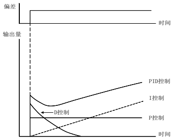
图 7-25 PID 控制的作用
