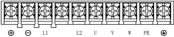
图 I HGD303 变频器主端子
