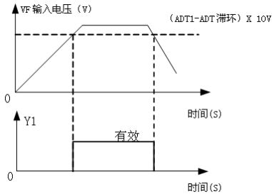
图 7-16 模拟量检测水平
