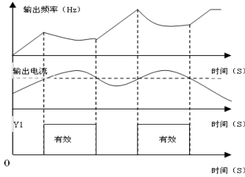
图 7-19 频率零速检测
