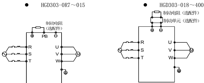
图 3-3 主回路标准接线
