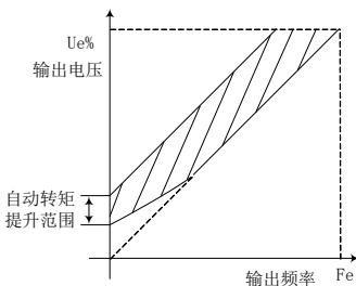
图 8-2 自动转矩提升
