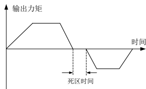
图 7-31 正/负力矩死区时间
