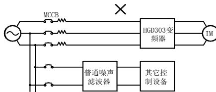
图 3-6 噪声滤波器的错误安装
