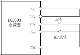
（a）F0.05=0 两线控制接线示意图
