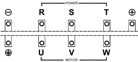
(c) 90kW 及以上规格主回路端子
