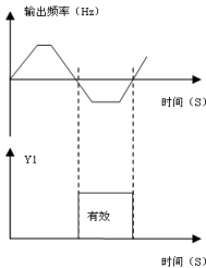
图 7-12 变频器正反转
