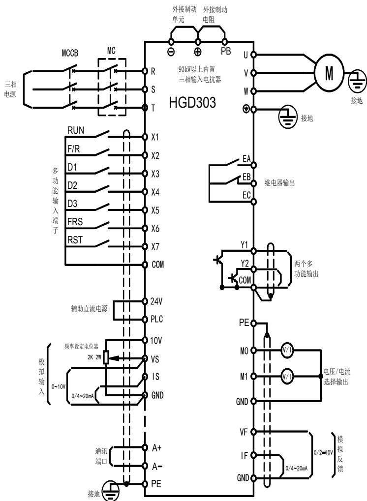
图 3-18 控制回路端子连接图
