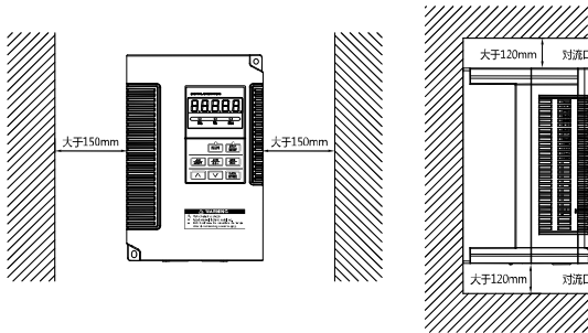
图 2-2 变频器安装方向和空间
