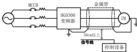
图 3-8 感应干扰对策
