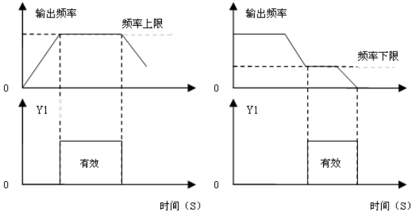
图 7-14 频率输出上下限到达
