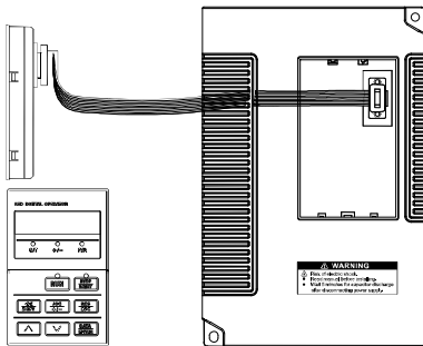
图 3-19 拉出键盘装延长线
