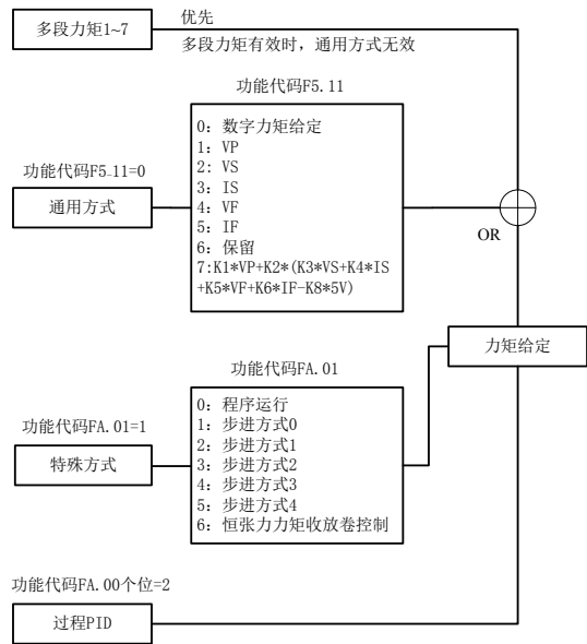
图 1-2 力矩输入方式示意图
