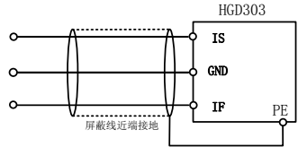
图 3-13 IS/IF 端子配线图
