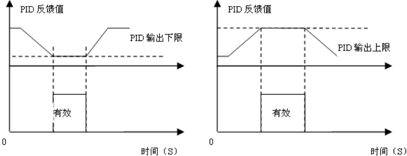
图 7-15 PID 反馈上下限
