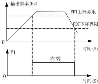
图 7-21 频率输出水平 FDT
