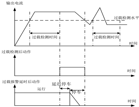
图 7-17 过载预警输出
