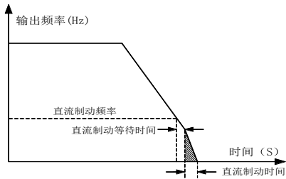
图 7-23 停车直流制动过程
