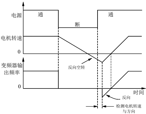
图 7-5 转速追踪启动
