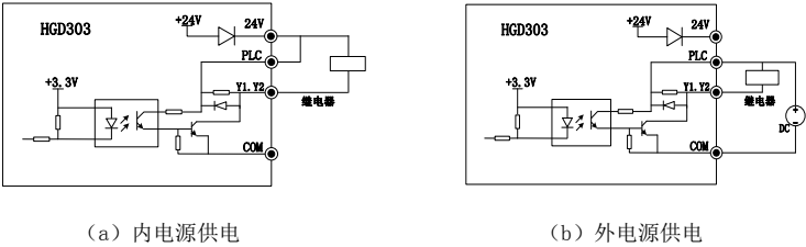
图 7-8 可编程端子供电方式
