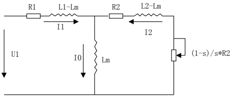
图 7-7 异步电动机稳态等效模型
