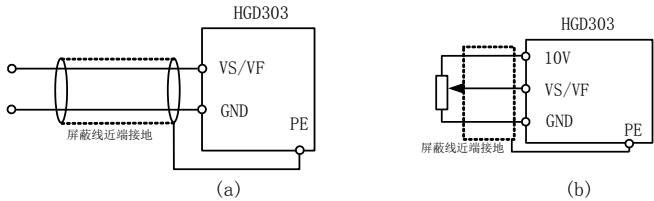
图 3-12 VS/VF 端子配线图
