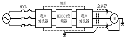
图 3-9 射频干扰对策
