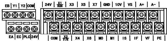
图 3-11 控制回路端子排列
