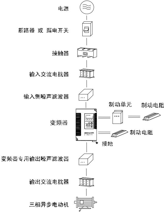
图 3-1 变频器与外围设备的连接图
