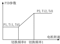
图 7-29 PID 参数示意图
