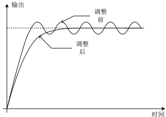
图 7-28 抑制输出周期振荡
