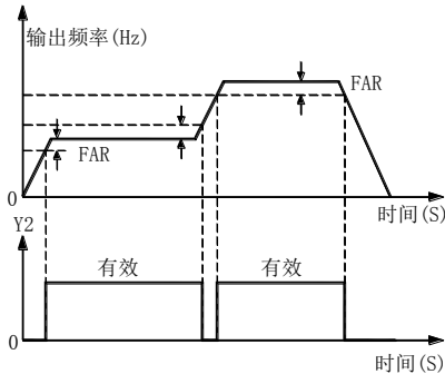
图 7-11 输出频率范围 FAR
