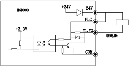
图 3-14 (a) 多功能输出端子用内部电源接线方式
