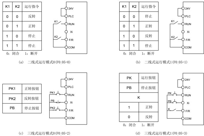
图 1-3 端子运行方式控制逻辑图
