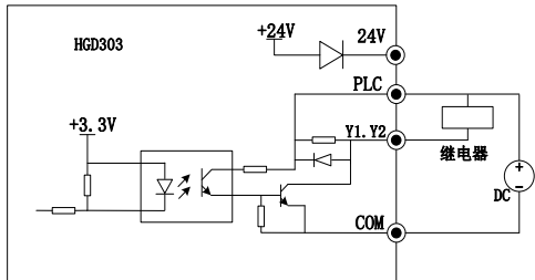
图 3-14 (b) 多功能输出端子用外部电源接线方式
